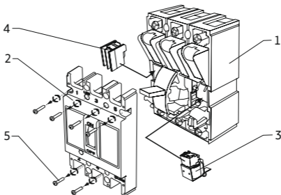
Рисунок 2 - Установка дополнительных устройств.
